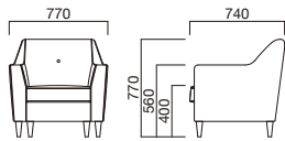
FN009-77 W770 D740 H770 (SH400 AH560) mm 上部:ウレタンフォーム 脚部:ホワイトアッシュ材 ボタン締め1つ rank1 ¥158,000 rank4 ¥191,000 rank2 ¥169,000 rank5 ¥202,000 rank3 ¥180,000
