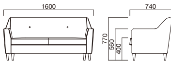
FN009-160 W1600 D740 H770 (SH400 AH560) mm 上部:ウレタンフォーム 脚部:ホワイトアッシュ材 ボタン締め2つ rank1 ¥221,000 rank4 ¥260,000 rank2 ¥234,000 rank5 ¥273,000 rank3 ¥247,000
