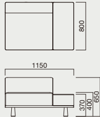
FN112-115R 1Pソファ+ファブリックテーブル W1150 D800 H650 (SH400) mm rank1 ¥213,000 rank4 ¥231,000 rank2 ¥219,000 rank5 ¥237,000 rank3 ¥225,000
