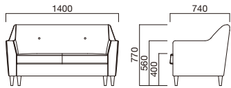
FN009-140 W1400 D740 H770 (SH400 AH560) mm 上部:ウレタンフォーム 脚部:ホワイトアッシュ材 ボタン締め2つ rank1 ¥206,000 rank4 ¥242,000 rank2 ¥218,000 rank5 ¥254,000 rank3 ¥230,000
