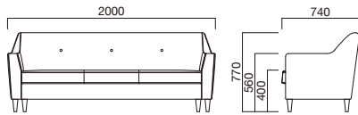
FN009-200 W2000 D740 H770 (SH400 AH560) mm 上部:ウレタンフォーム 脚部:ホワイトアッシュ材 ボタン締め3つ rank1 ¥259,000 rank4 ¥304,000 rank2 ¥274,000 rank5 ¥319,000 rank3 ¥289,000
