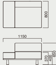
FN112-115L 1Pソファ+ファブリックテーブル W1150 D800 H650 (SH400) mm rank1 ¥213,000 rank4 ¥231,000 rank2 ¥219,000 rank5 ¥237,000 rank3 ¥225,000
