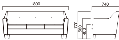
FN009-180 W1800 D740 H770 (SH400 AH560) mm 上部:ウレタンフォーム 脚部:ホワイトアッシュ材 ボタン締め3つ rank1 ¥244,000 rank4 ¥286,000 rank2 ¥258,000 rank5 ¥300,000 rank3 ¥272,000
